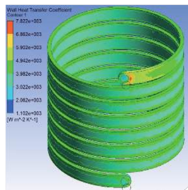
ウォータージャケットの流れを 最適化する冷却設計
