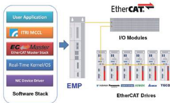
オールデジタルのモーションコントロールプラットフォームの構造（EMP）
